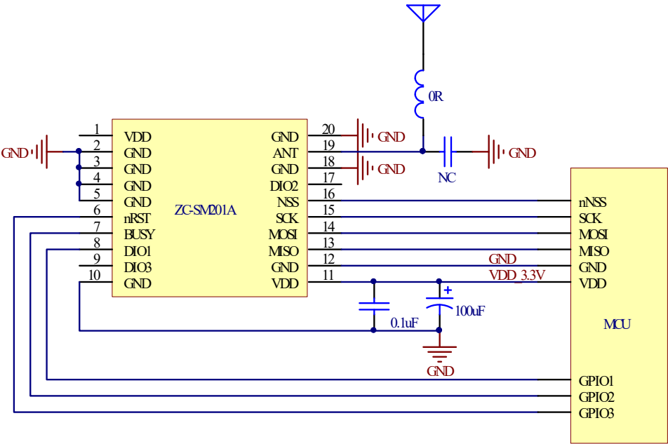
图 4 模组应用参考设计
