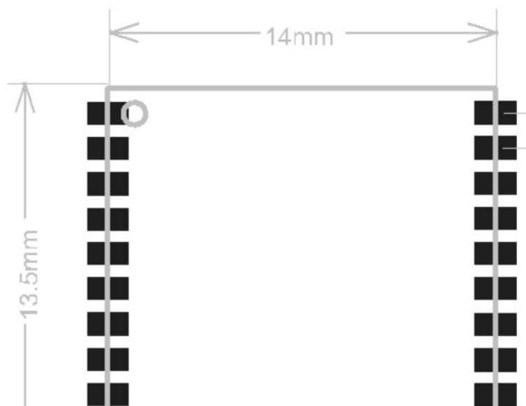
图 5 模组 PCB 封装尺寸
