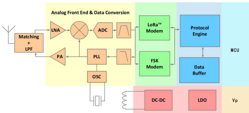
图 1 无线收发芯片架构图
