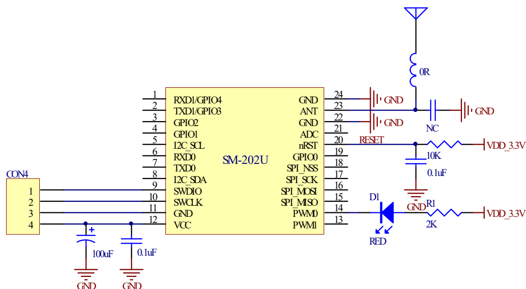
图 4 模组应用参考设计
